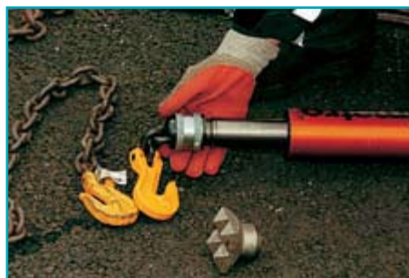
Гидроцилиндр с подтягивающей насадкой (не все гидроцилиндры могут тянуть)
