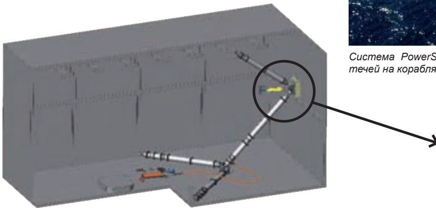
Закрытие течи в переборке при помощи гидравлического комплекта ликвидации течей PowerShore™.
